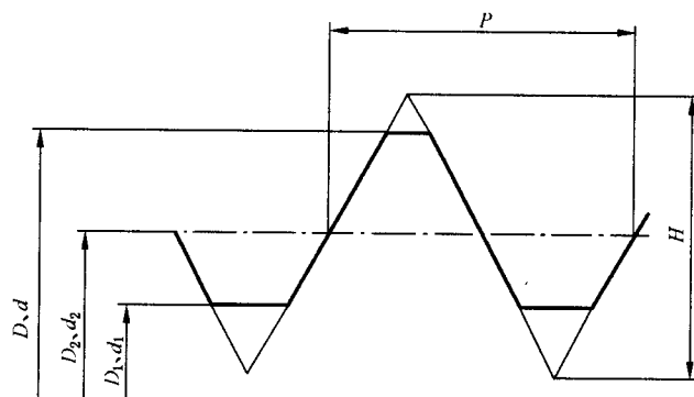
图 1 基本尺寸
